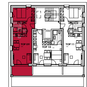
Grundriss 3 OG_Haus 4
